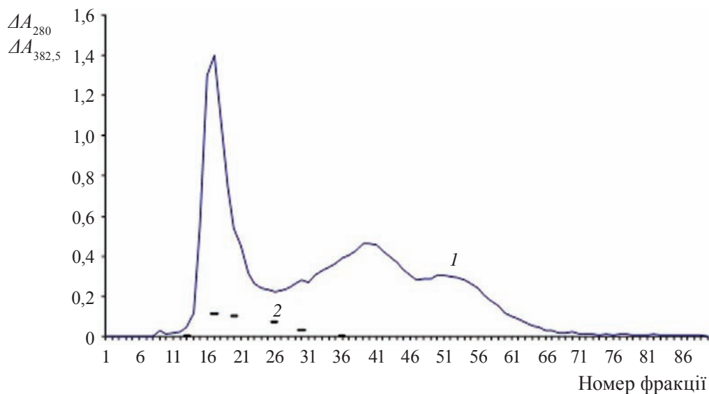
Рис. 1. Профіль елюції гель-фільтрації на сефадексі G-100 висоленої сульфатом амонію 3,0 М фракції, що містить пептидгідролазу личинок дрозофіли: 1 – піки розподілу протеїну, 2 – лінія розподілу ензимної активності
