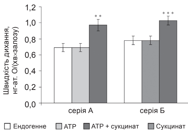
Рис. 2. Дихання суспензії ізольованих слинних залоз личинки дзвінця після пермеабілізації плазматичної мембрани секреторних клітин за допомогою АТР: А – АТР вносили перед сукцинатом; Б – першим вносили сукцинат, а потім АТР; [АТР] = 100 мкМ, [сукцинат] = 0,35 мМ, [Ca^{2+}]_e = 1,76 мМ; ** різниця щодо ендогенного дихання статистично вірогідна з P \leq 0,01 , *** P \leq 0,001 ; n = 5
