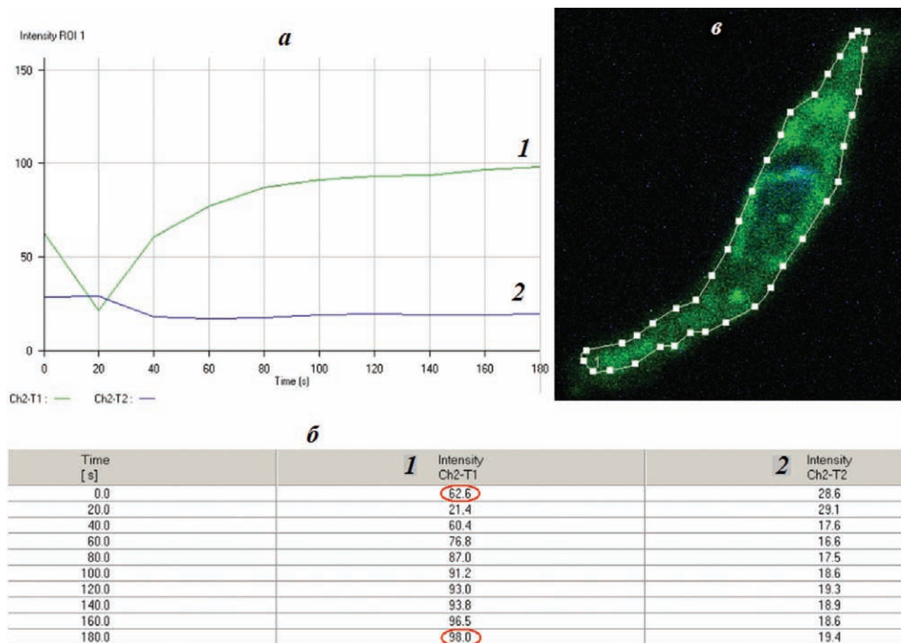
Рис. 5. Збільшення інтенсивності флуоресценції міоцита, попередньо навантаженого \text{DiOC}_6(3) , за внесення 100 нМ С-99 у присутності 1 мМ убаїну. Результати характерного дослід: а – кінетика спалаху флуоресценції \text{DiOC}_6(3) (крива 1) після внесення С-99, крива 2 – інтенсивність флуоресценції ядерного барвника Hoechst 33342; б – цифрова презентація графічних результатів а (1 – \text{DiOC}_6(3) , 2 – Hoechst 33342); результати (а) і (б) одержані на основі оцінювання інтенсивності флуоресценції, усередненої за площиною оптичного зрізу міоцита (в), параметр ROI 1
