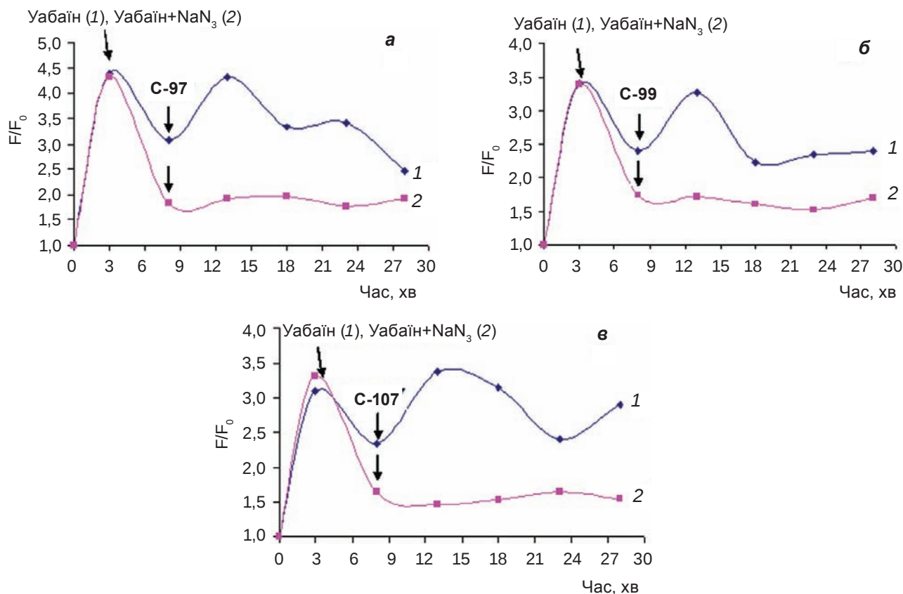
Рис. 4. Дія калікс[4]аренів С-97, С-99, С-107 та С-150 на поляризацію внутрішньої мітохондріальної мембрани. Стрілочкою вказано момент додавання (на 3-й хв інкубації клітин із зондом) 1 мМ убаїну (1) або 1 мМ убаїну + 5 мМ \text{NaN}_3 (2) та (на 8-й хв) каліксаренів (100 нМ). Результати характерного дослід. Флуоресцентний зонд – 100 нМ \text{DiOC}_6(3)
