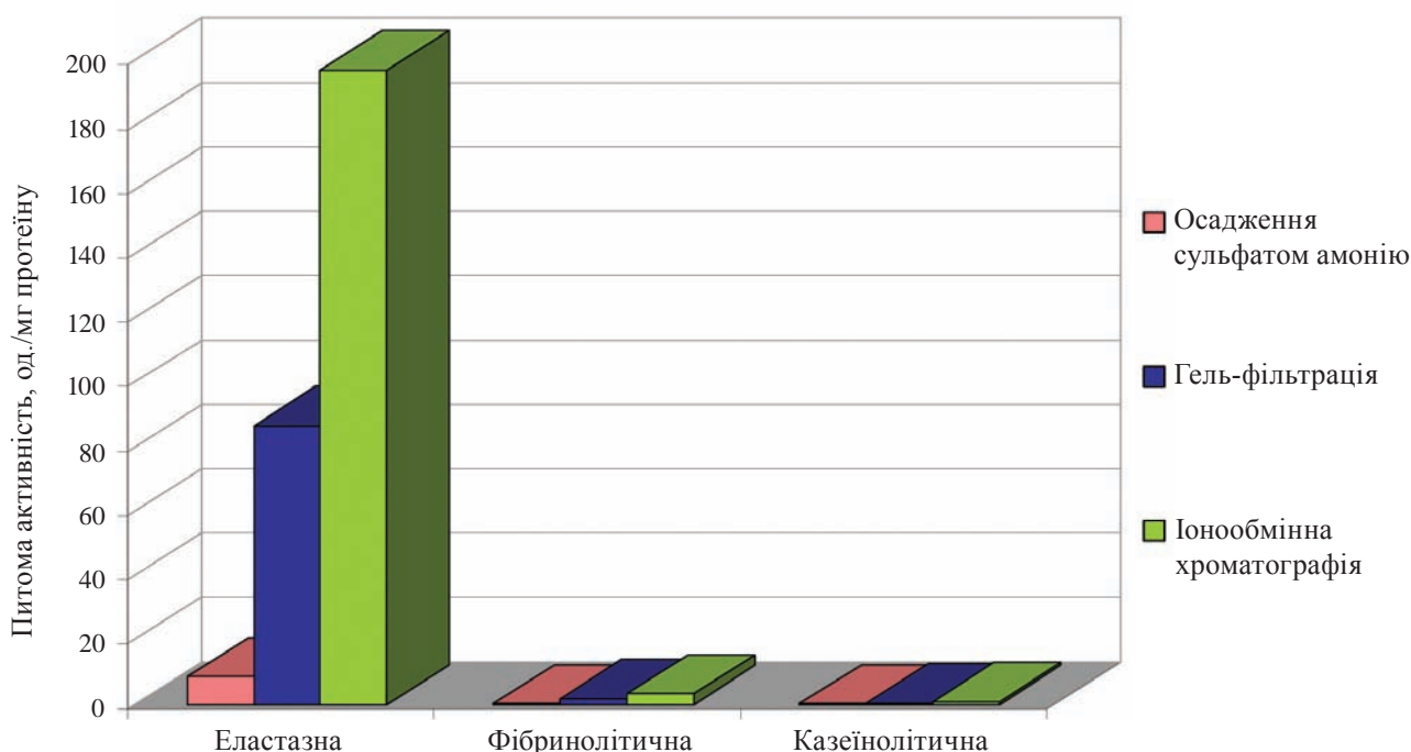
Рис. 2. Спектр активності пептидази різного ступеня очищення
