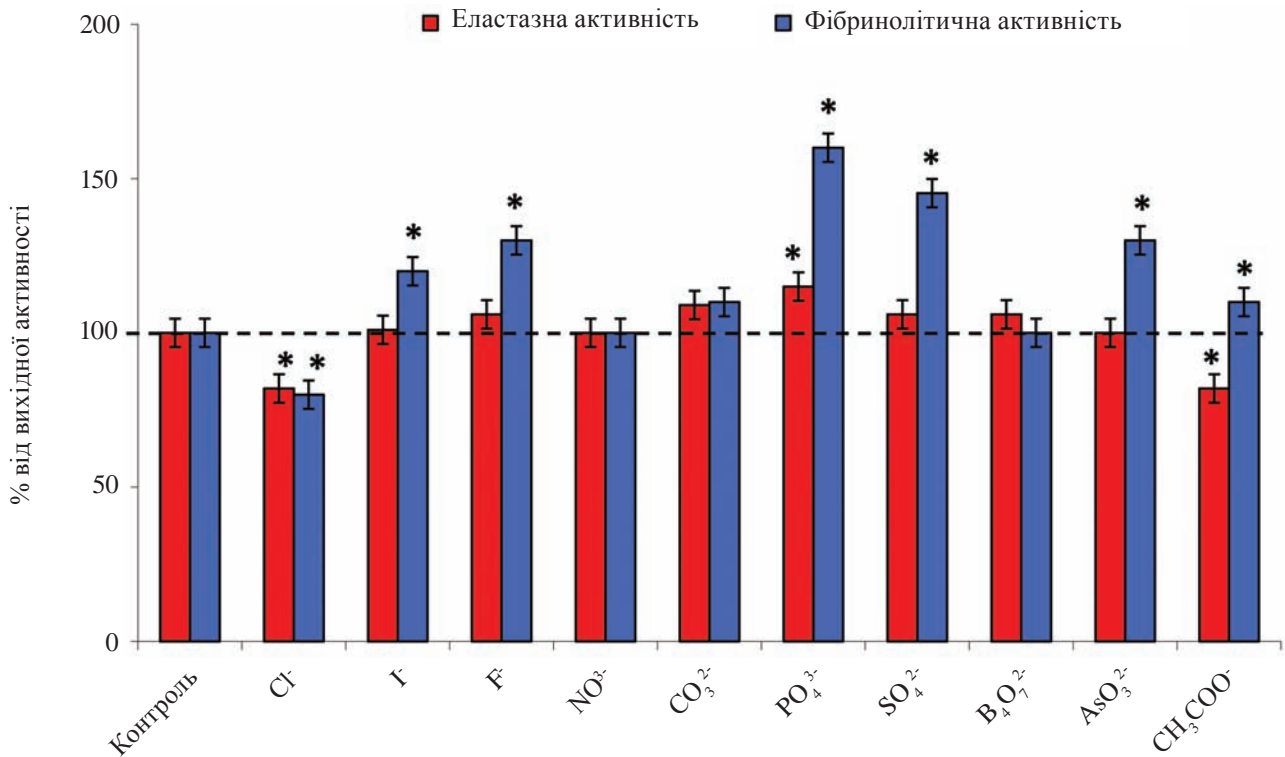
Рис. 10. Вплив аніонів на активність пептидази B. thuringiensis IMB B-7324 (* P \leq 0,05 порівняно з контролем, n = 5 )
