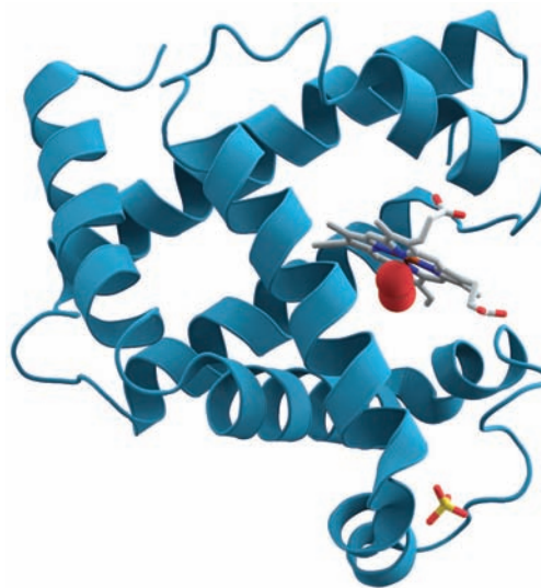
Модель міоглобіну [51]
